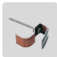
Euro-clip pour faîtière demi- ronde et plate
